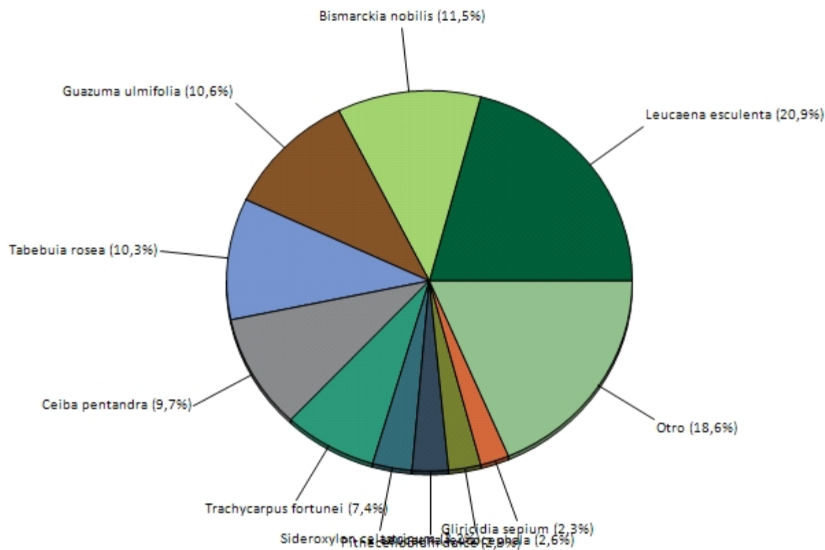
Figura 1. Composición de las especies de árboles en Parque Chiapasionate
