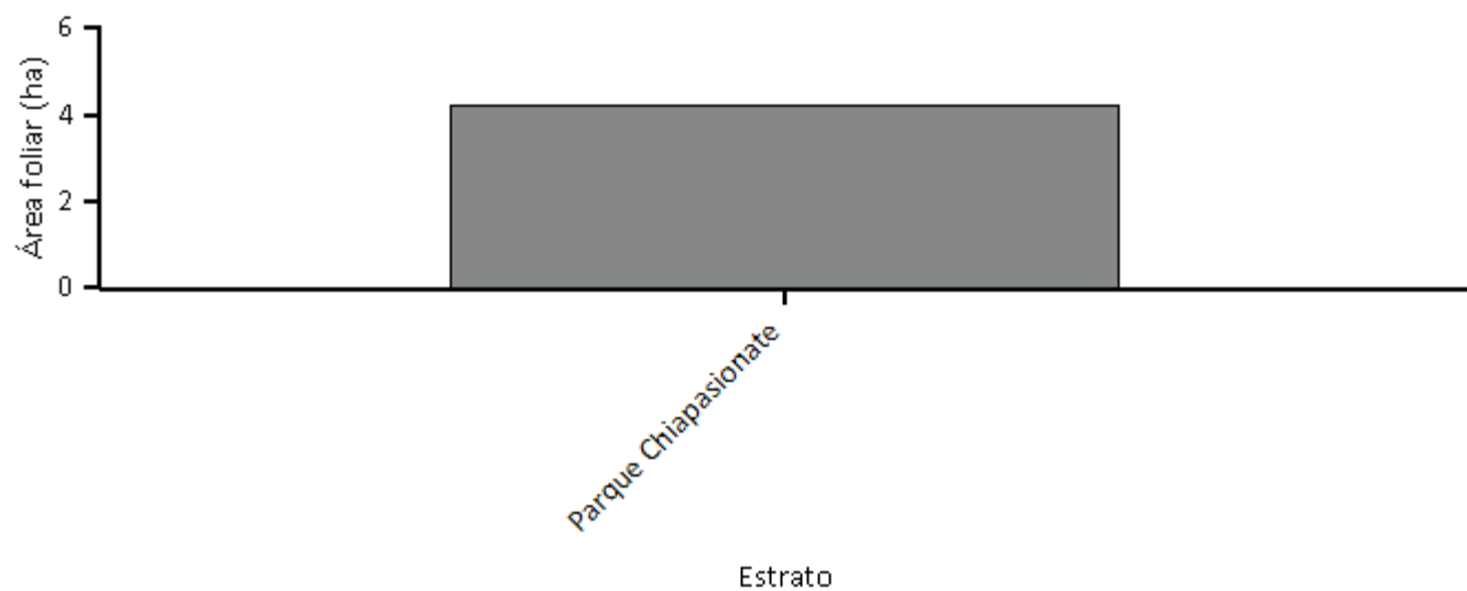
Figura 5. Área de las hojas por estrato, Parque Chiapasonate
