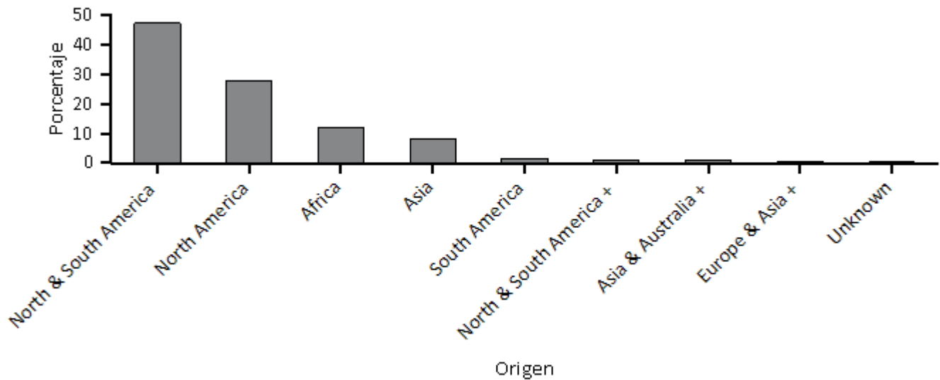
Figura 4. Porcentaje de la población de árboles vivos por área de origen, Parque Chiapasionate
