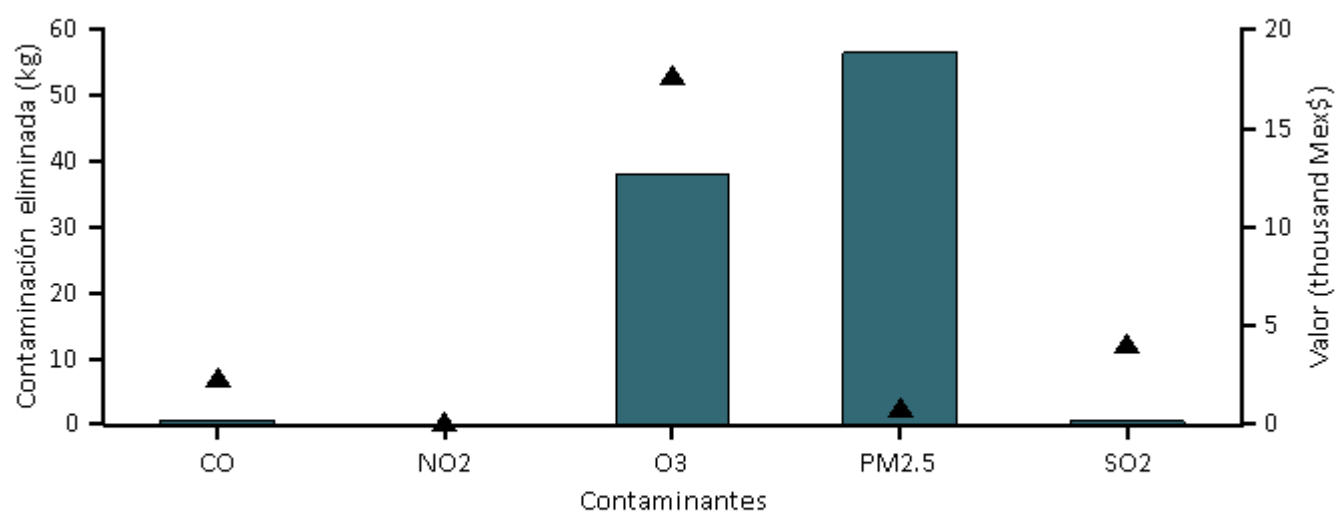
Figura 7. Eliminación anual de la contaminación (puntos) y valor (barras) por árboles urbanos, Parque Chiapasionate
