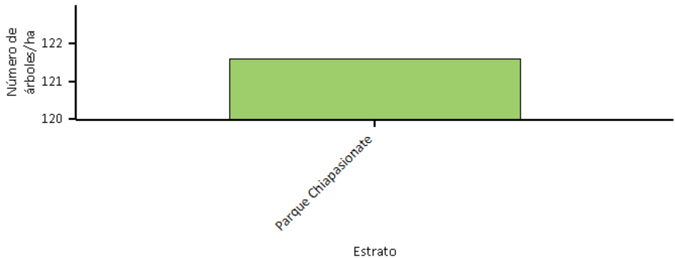
Figura 2. Número de árboles/ha en Parque Chiapasonate por estrato
