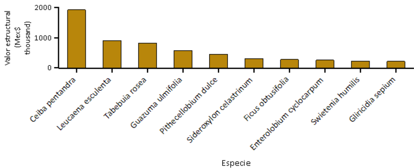
Figura 11. Especies de árboles con el mayor valor estructural, Parque Chiapasionate
