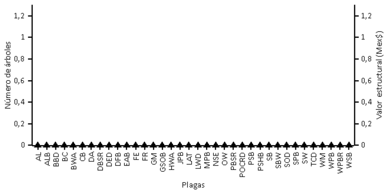
Figura 12. Número de árboles en riesgo (puntos) y valor de compensación relacionado (barras) por posibles plagas, Parque Chiapasionate
